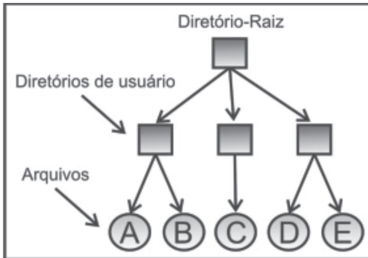
Figura 56: Projeto de sistemas de arquivos com dois níveis.
