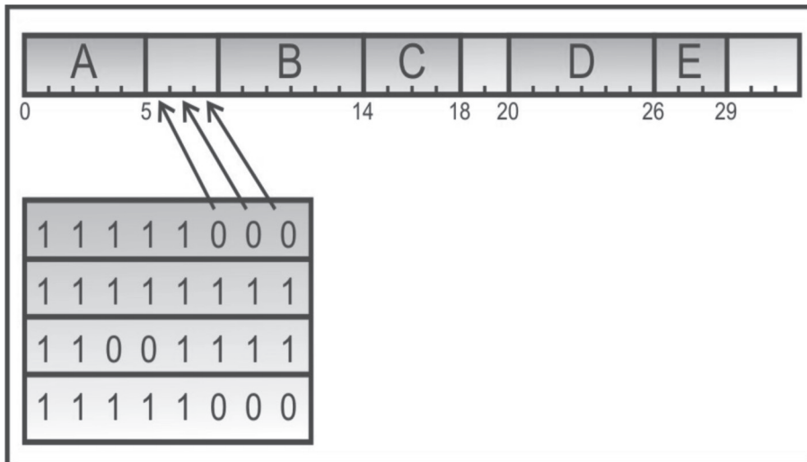
Figura 41: Memória dividida em unidade de alocação e o Mapa de bits correspondente.
