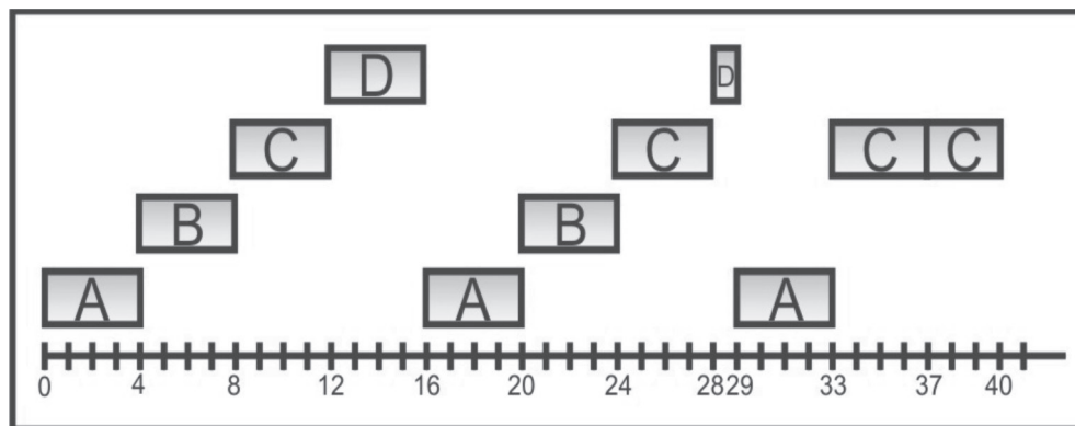
Figura 21: Diagrama de tempo usando a política Round Robin (quantum 4 unidades de tempo).
