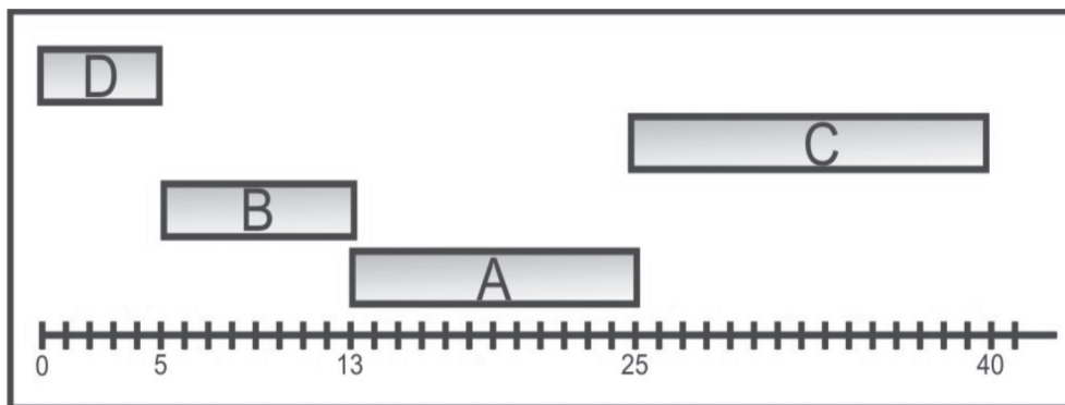
Figura 22: Diagrama de tempo usando a política por prioridades.
