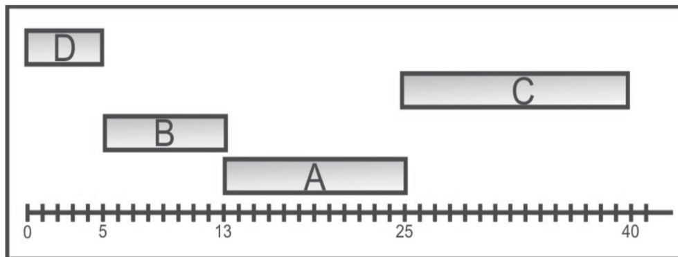
Figura 20: Diagrama de tempo usando a política Menor Tarefa Primeiro.
