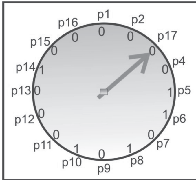
Figura 49: Seleção de página segundo o algoritmo de substituição de página do relógio
