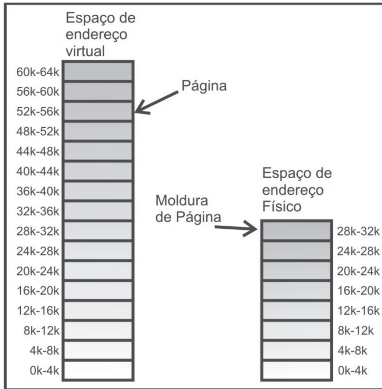
Figura 44: Técnica de paginação
