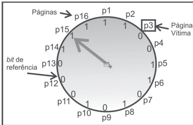
Figura 48: Algoritmo de substituição de página do relógio
