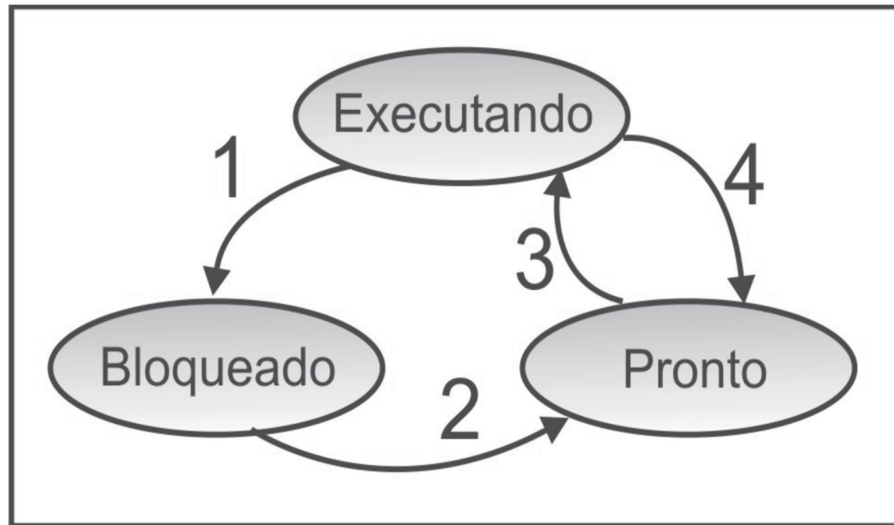
Figura 12: Transições possíveis entre os estados de um processo.
