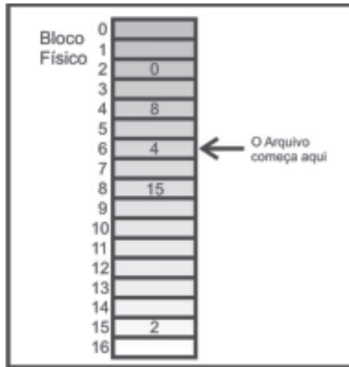
Figura 54: Implementação de arquivos por alocação por lista encadeada, utilizando índice.
