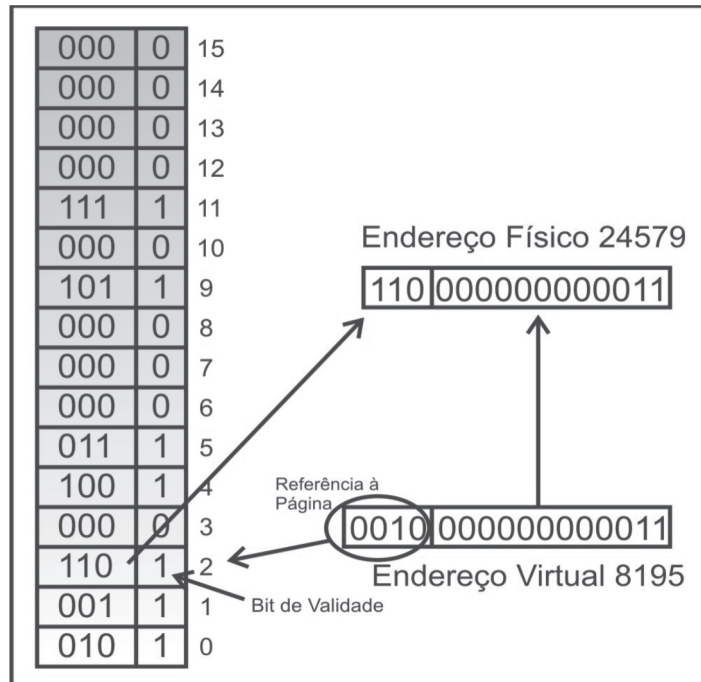
Figura 46: Mapeamento de endereço virtual para endereço físico
