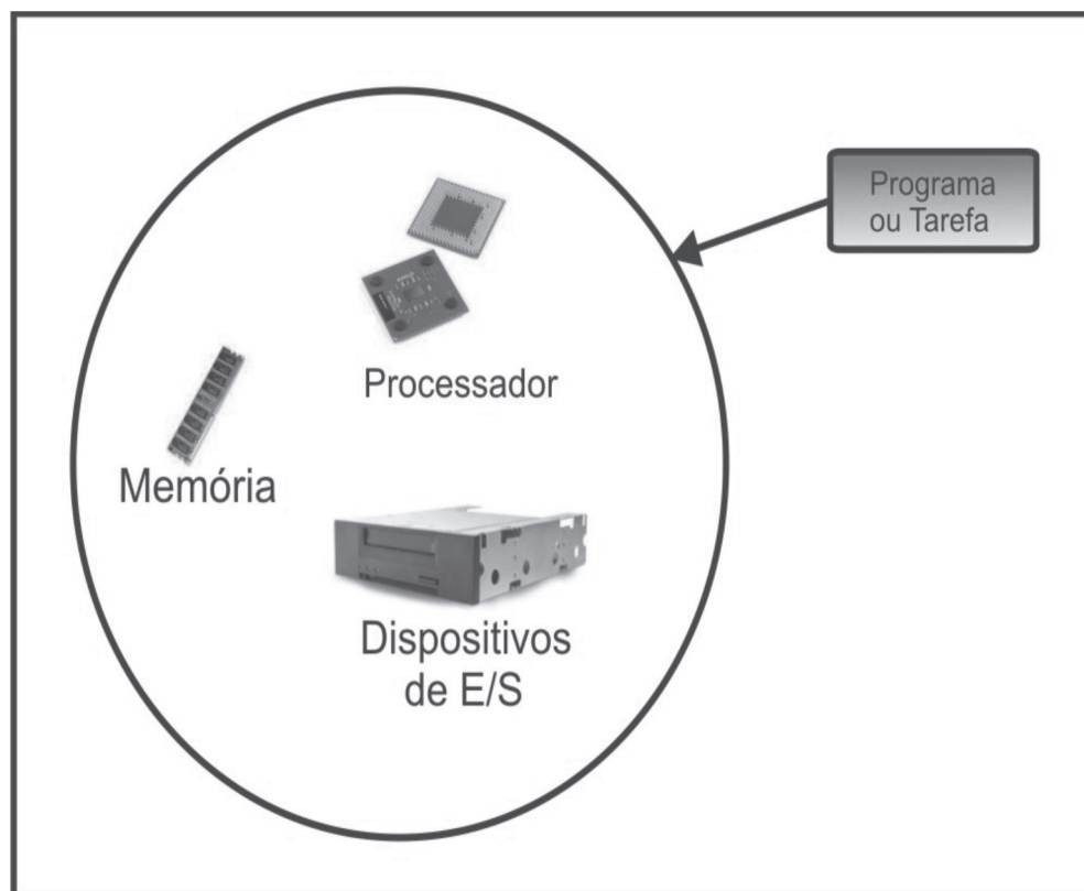
Figura 9: Sistemas monoprogramáveis.
