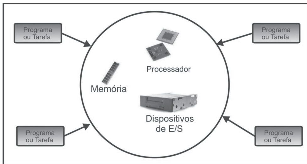
Figura 10: Sistemas Multiprogramáveis.
