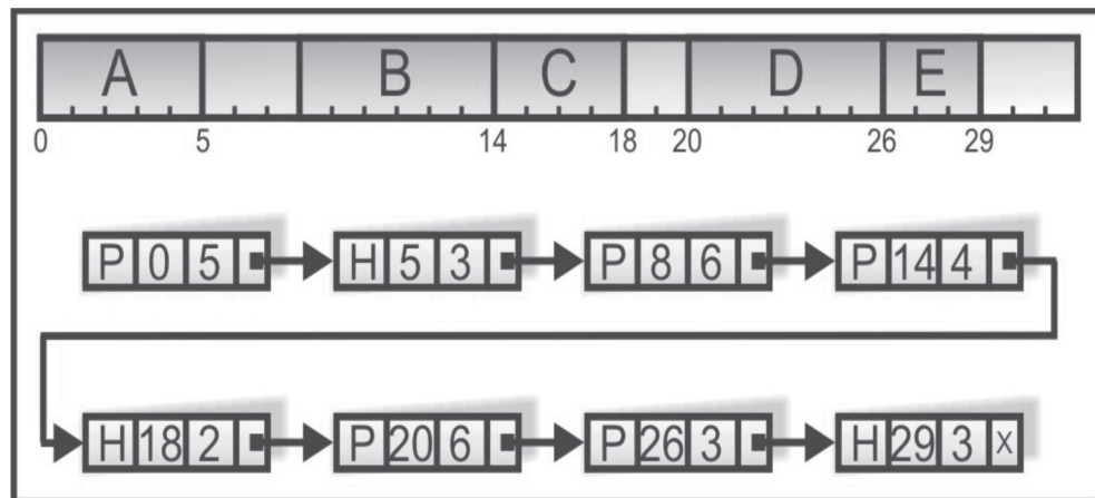
Figura 42: Memória dividida em unidade de alocação, monitorada através de lista encadeada.
