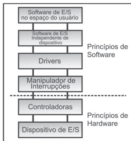
Figura 23: Princípios de hardware e de software de E/S.
