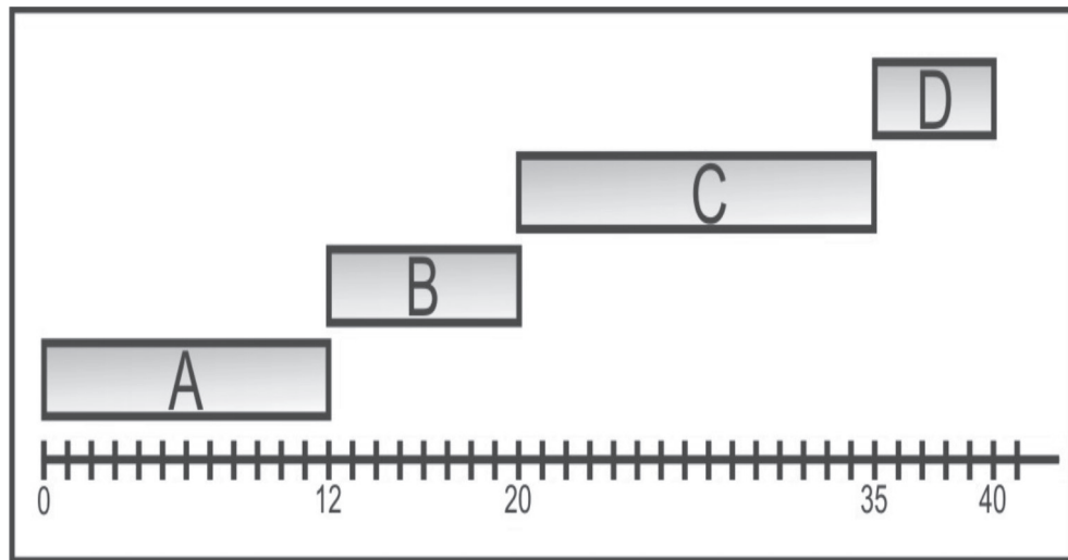
Figura 19: Diagrama de tempo usando a política FIFO.
