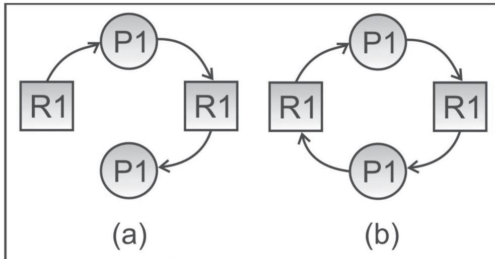
Figura 27: Modelagem através de grafos. (a) Situação onde não está caracterizado deadlock . (b) situação onde se caracteriza um deadlock .
