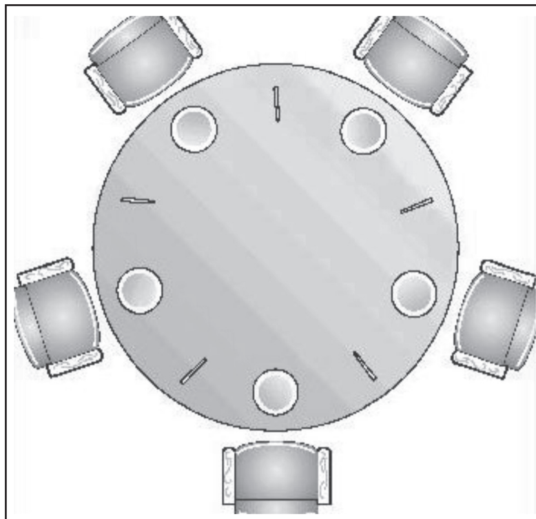
Figura 17: O problema clássico de comunicação interprocessos do Jantar dos Filósofos.
