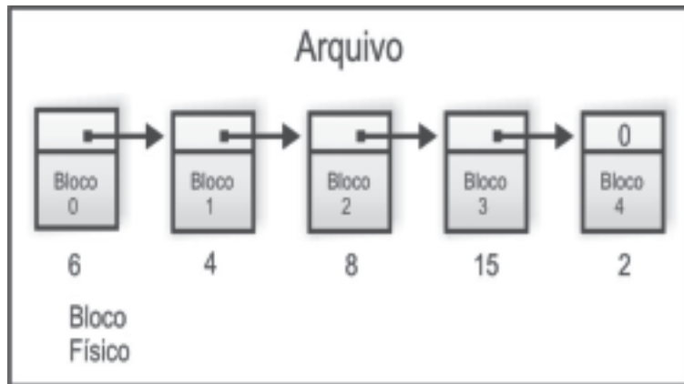
Figura 53: Implementação de arquivos por alocação por lista encadeada.
