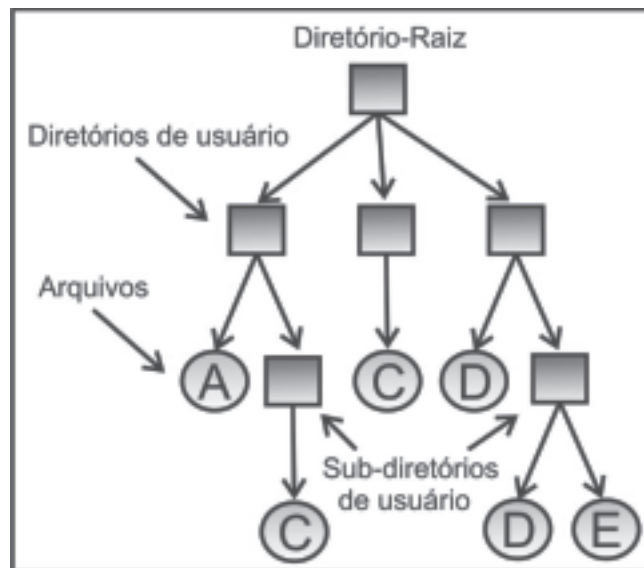
Figura 57: Projeto de sistemas de arquivos hierárquico.
