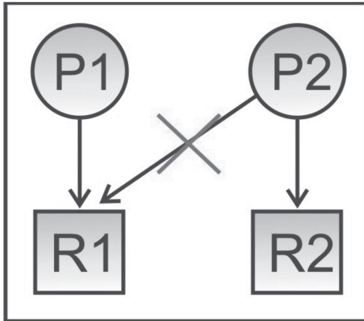
Figura 29: Recursos ordenados numericamente
