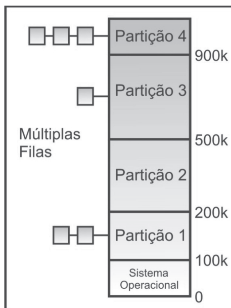
Figura 38: Esquema de gerência de memória para multiprogramação com partições fixas.
