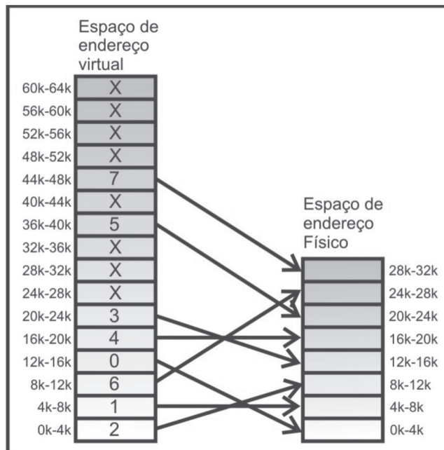
Figura 45: Mapeamento da memória virtual.
