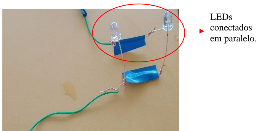
Figura 10: Associação de LEDs em Paralelo, ligados por um interruptor com uma tensão de 3 V.
