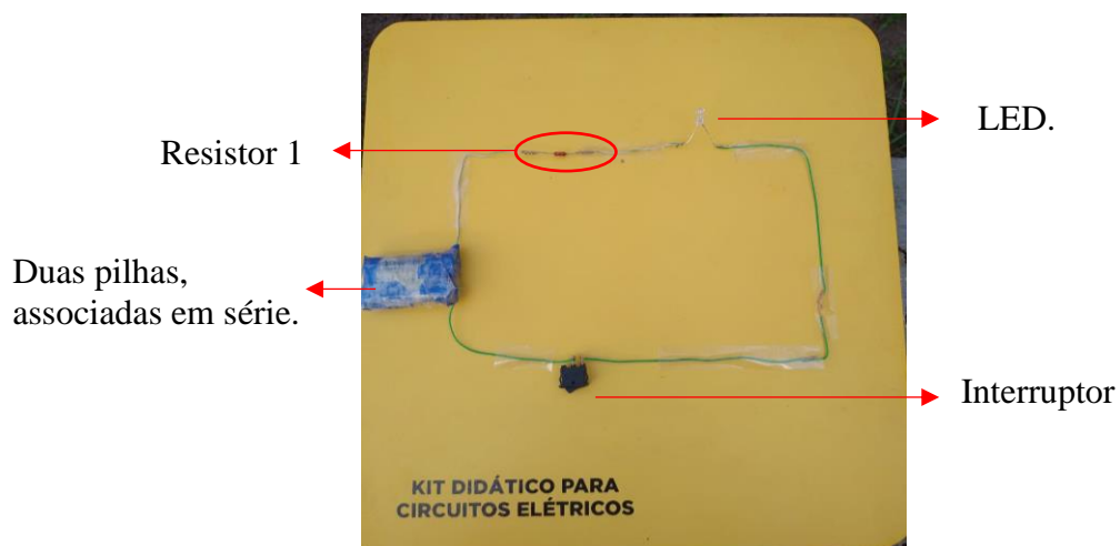
Figura 8 – Aparato final do experimento 2, circuito simples com um interruptor e um LED e um resistor.
