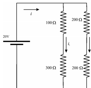
Figura 8 - Circuito composto por resistores mistos, alimentado por uma bateria de tensão 20 V.
