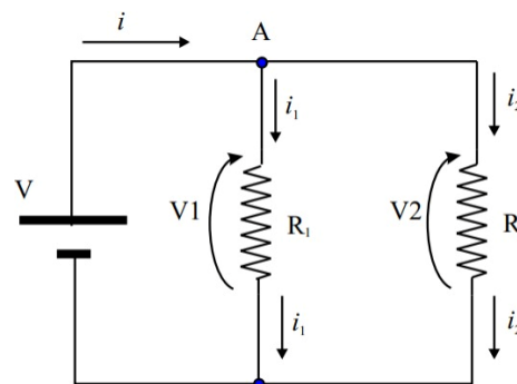
Figura 7 - Circuito composto por dois resistores em paralelo, e uma bateria de tensão V.
