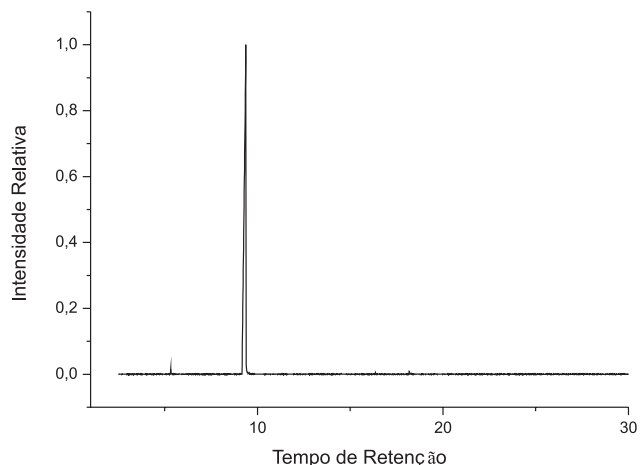
Figura 2. Perfil cromatográfico (TIC) do óleo essencial de Croton zehntneri
