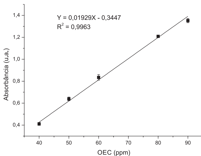
Figura 4. Curva de Calibração do óleo essencial de Croton zehntneri
