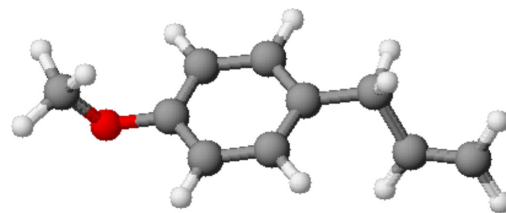
Figura 1. Estrutura do estragol (modelo bolas e vareta), principal constituinte do óleo essencial de Croton zehntneri , otimizada em programa ACD/3D: ChemSketch
