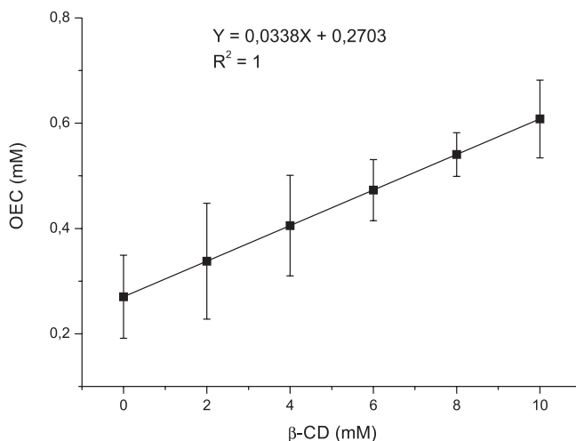
Figura 5. Diagrama de solubilidade do óleo essencial de Croton zehntneri em presença de \beta -ciclodextrina ( \beta -CD)
