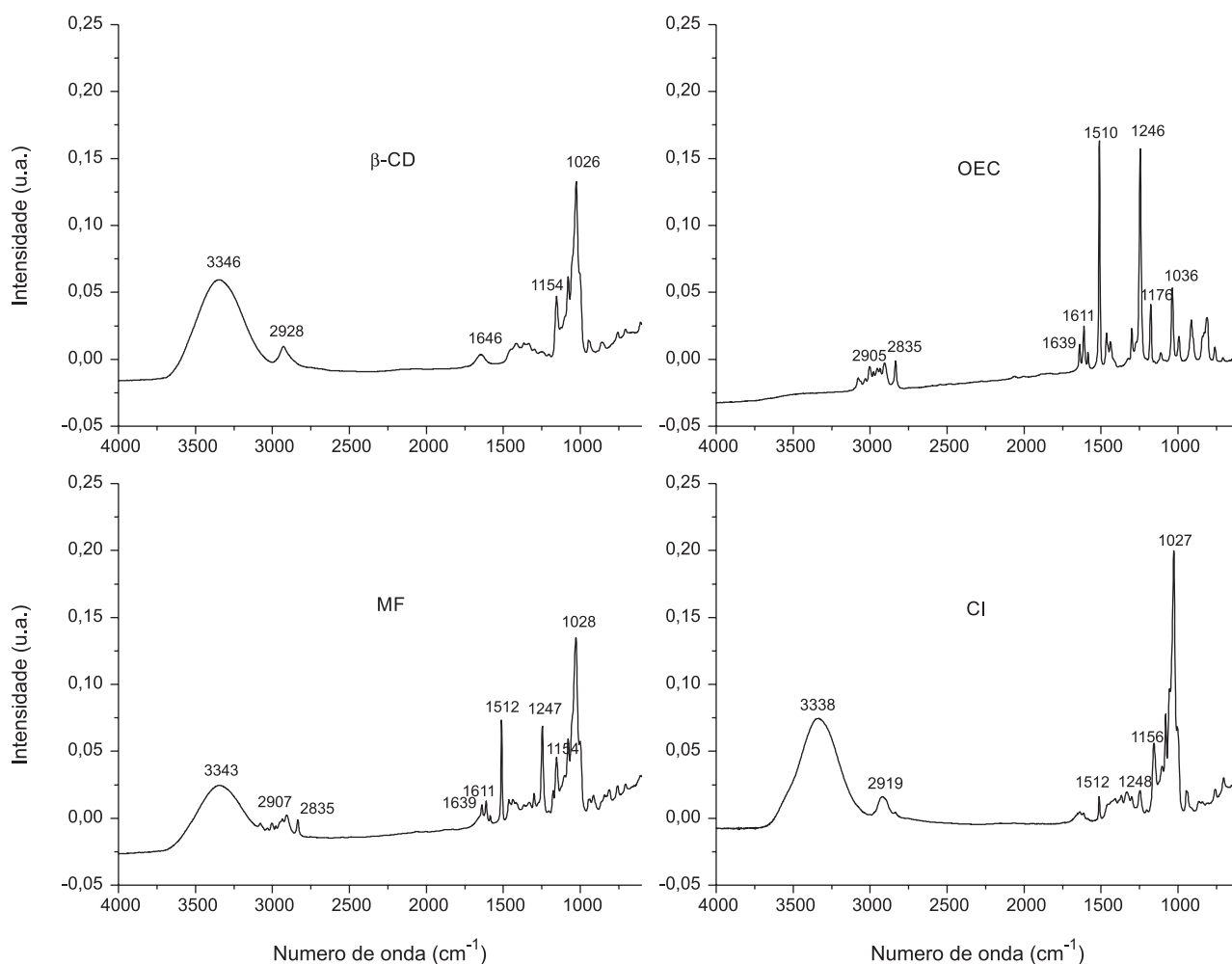
Figura 6. Espectros de Infravermelho das Amostras de \beta -ciclodextrina ( \beta -CD), Mistura Física (MF), Complexo de Inclusão (CI) e óleo essencial de Croton zehntneri (OEC)
