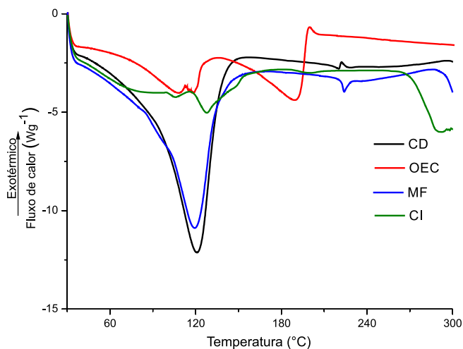
Figura 7. Termograma de DSC das Amostras de \beta -ciclodextrina ( \beta -CD), Mistura Física (MF), Complexo de Inclusão (CI) e óleo essencial de Croton zehntneri (OEC)
