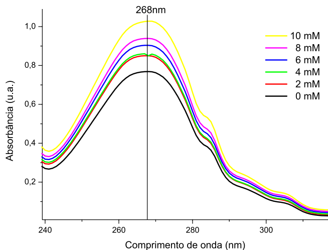
Figura 3. Leitura espectrofotométrica do óleo essencial de Croton zehntneri
